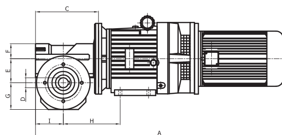
FORMA TYPE 41 Riduttore P085-P110 Gear-box P085-P110
