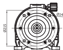
FORMA TYPE 11 ALBERO INGRESSO FEMMINA INPUT FEMALE SHAFT
